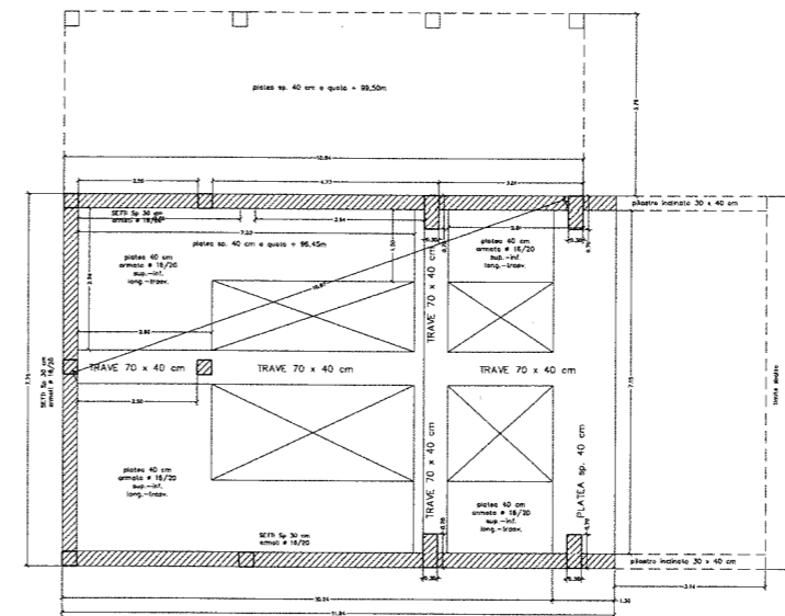
PIANTA IMPALCATO QUOTA m: 0.00 - 95.95 m.s.m.
