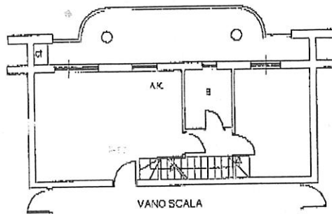
PIANO SECONDO H=ML 2,70
