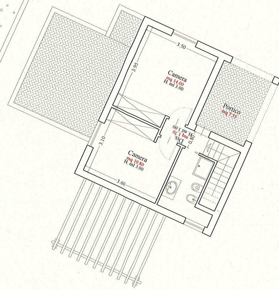
Piano Primo 1:100
